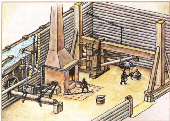
Тульская металлургическая мануфактура XVII в. Современная реконструкция
